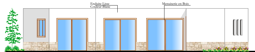
FACADE GAUCHE
