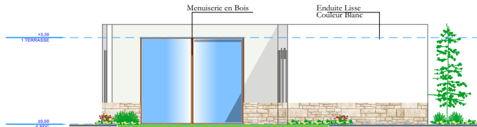
FACADE GAUCHE
