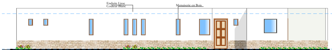
FACADE PRINCIPALE
